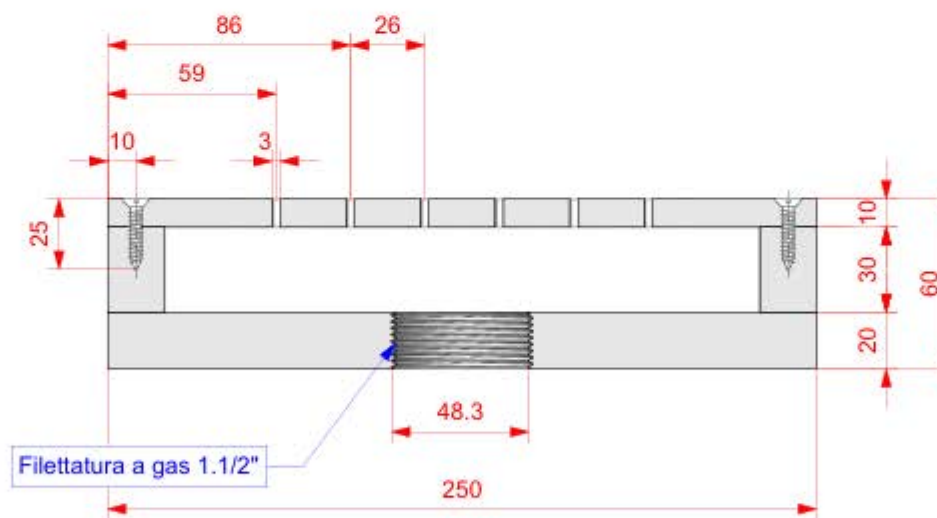
2 Sezione Scale: Half Actual Size
